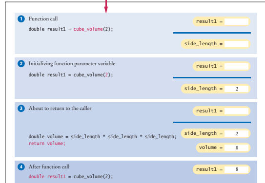
Figure 3 Parameter Passing
